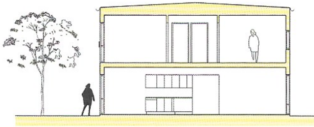
Sektion
